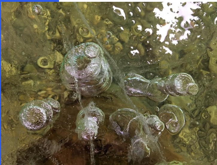
Methanblasen im Eis des Lunzer Sees ©Margaux Mathieu-Resuge
